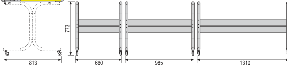
TROLLEY PER PLANET 2 GN 1/1
