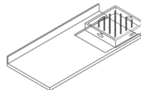
Ribasso per cestelli lavastoviglie
