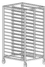
Carrelli per GN 2/1, 1/1, 15+15 file passo 85 mm
